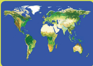
Distribución de las masas oceánicas y continentales
